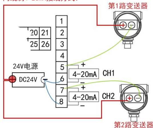
两线制4-20mA接线方式:
