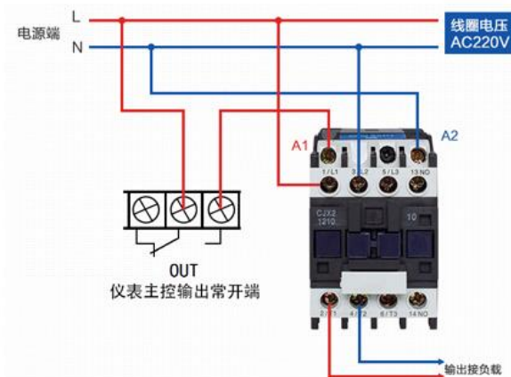
中间继电器接线方法
