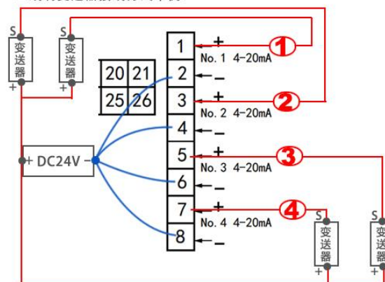
二线制变送器接线方式举例:
